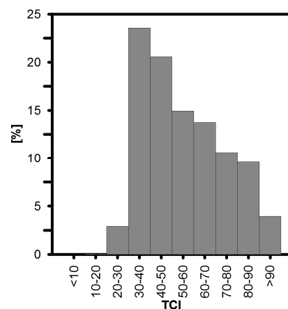
Rys. 2. Rozkład częstości wskaźnika TCI w Łodzi w latach 1966–2014
