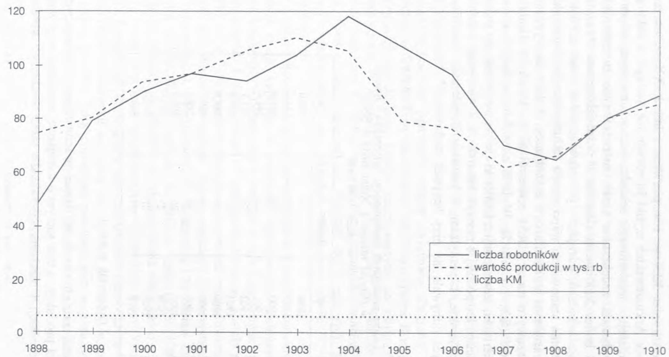
Wykres 1. Rozwój Fabryki Maszyn J. Arkuszewski w latach 1898-1910
