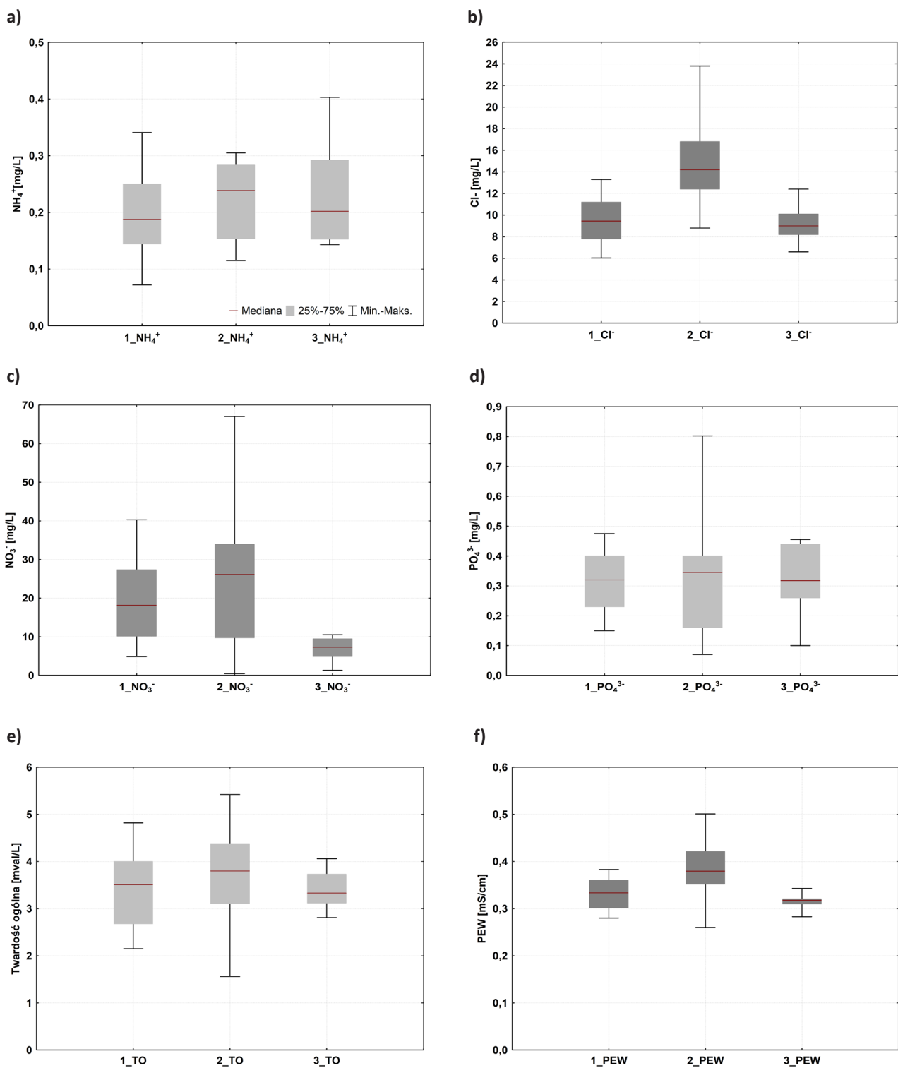
Rys. 3. Zakresy wybranych elementów hydrochemicznych w wodach grup źródeł badanych w latach 1996–2010; grupy hipsometryczne źródeł: 1 – górna, 2 – środkowa, 3 – dolna; a) jon amonowy, b) chlorki, c) azotany, d) ortofosforany, e) twardość ogólna, f) przewodność elektrolityczna właściwa
