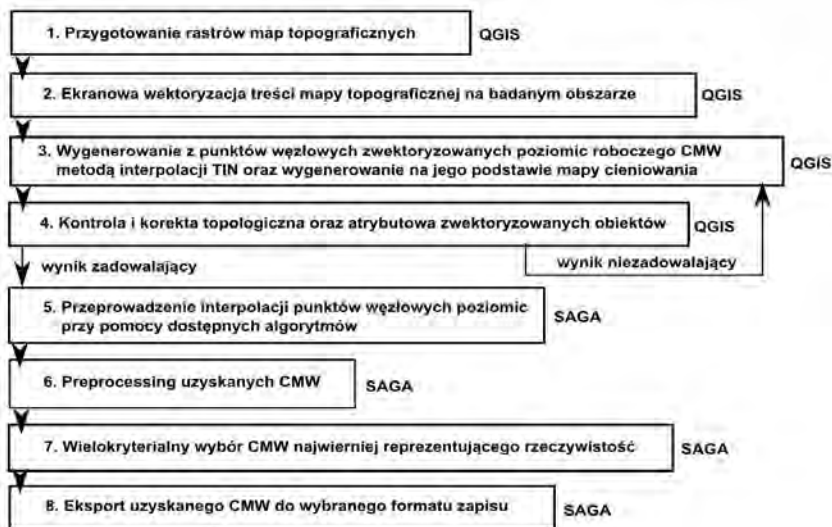
Rys. 1. Schemat postępowania prowadzącego do budowy CMW
