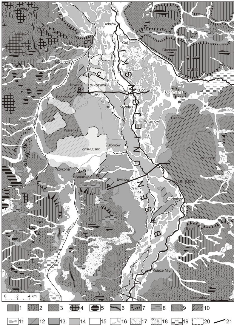
Ryc. 2. Szkic geomorfologiczny basenu uniejowskiego i jego otoczenia
