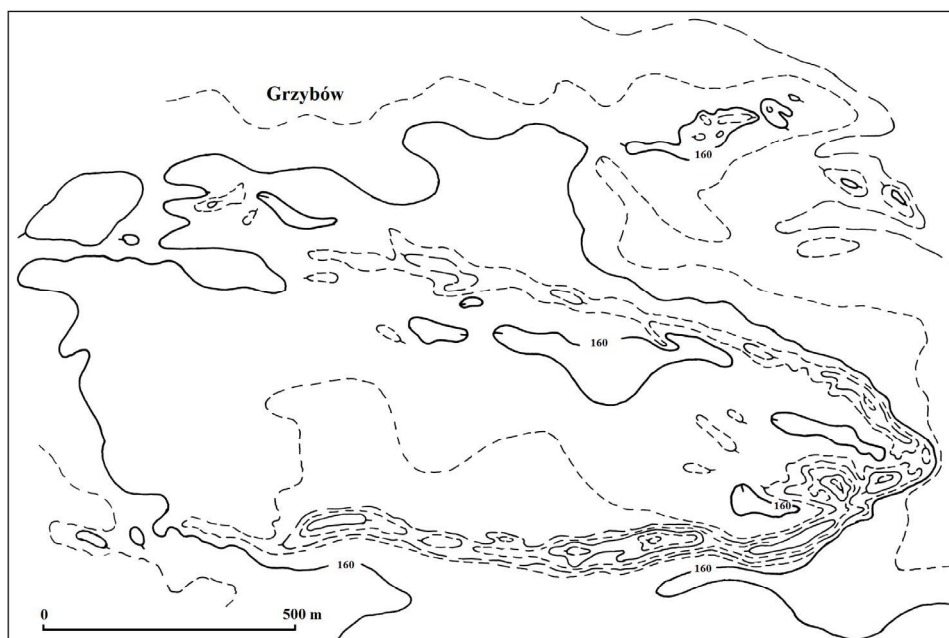
Ryc. 4. Wydma paraboliczna na południe od Grzybowa Źródło: opracowanie własne
