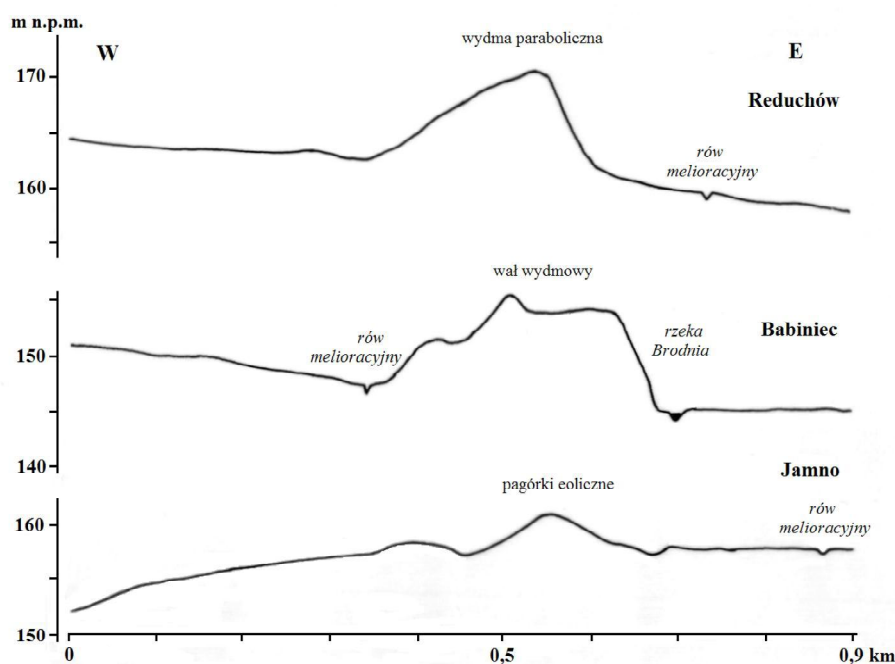
Ryc. 2. Rysunki poziomicowe wybranych wydm parabolicznych Źródło: opracowanie własne
