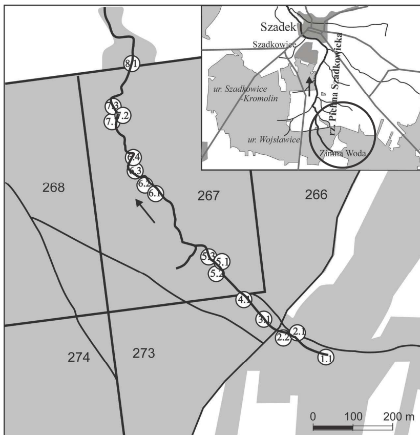
Ryc. 1. Teren badań. Rzeka Pichna Szadkowicka z zaznaczonymi punktami poboru prób Źródło: opracowanie własne
