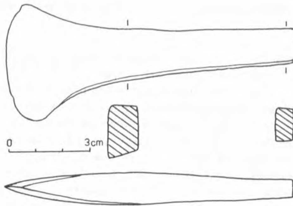
Rys. 1. Woźuczyn, woj. Zamość. Siekierka miedziana. L : B_1 = 2,5 ; B_1 : B_2 = 3,6 . Rys. A. Zakościelna
