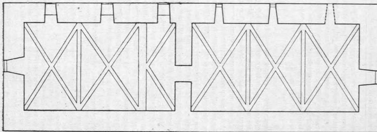
Rys. 6. Rekonstrukcja fazy gotyckiej
