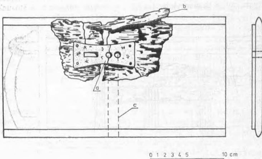
Rys. 2. Wieczko skrzyneczki
