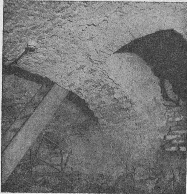
Fot. 3. Ostromecko, „pałac stary”, relikty muru starszego dworu w dolnej partii ściany pomieszczenia piwnicznego nr IV. Sklepienie kolebkowe z XVIII w. Fot. M. Sowińska, 6488/31/1976
